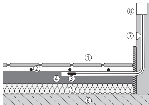
Abb. 1: Bodenkonstruktion (Beispiel)
