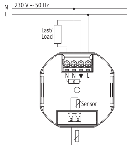
Abb. 3: Schaltbild x-net +e Unterputzregler 230 V
